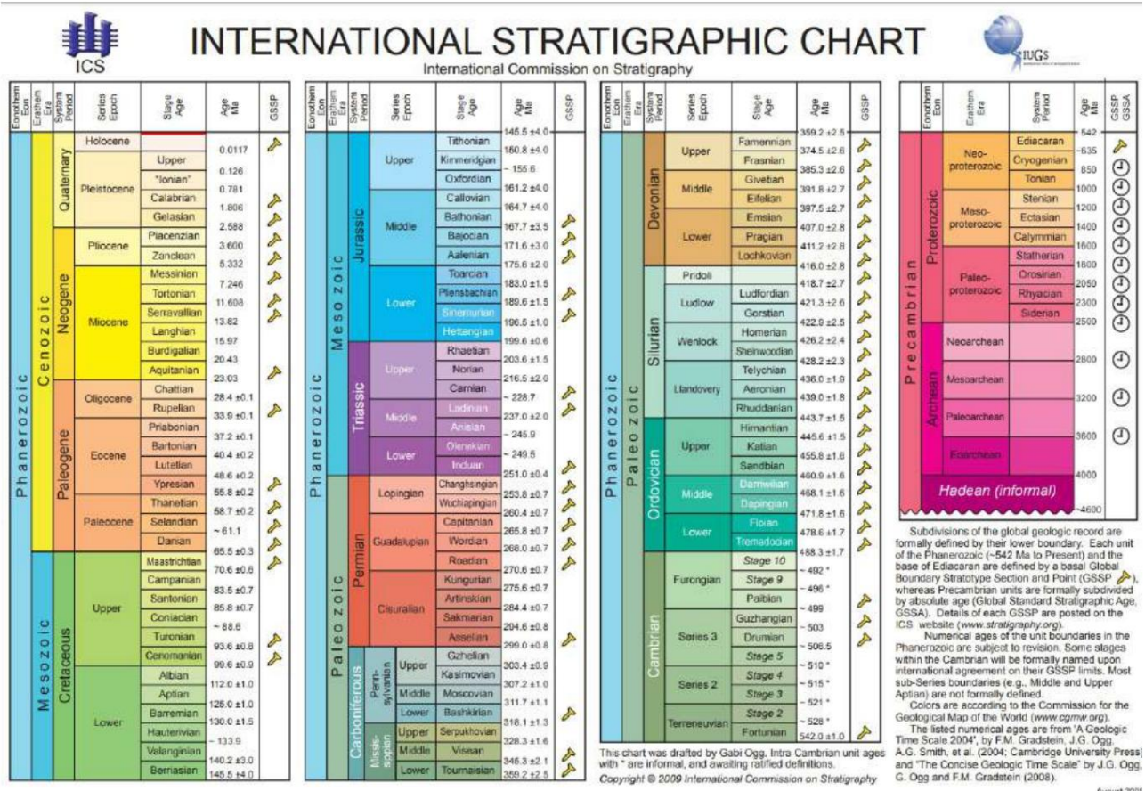
Figure 6. Carte stratigraphique géologique pour toute l'histoire géologique de la planète Terre. L'époque moderne est indiquée par la fine ligne rouge en haut de la colonne de gauche. Veuillez noter que l'échelle de temps est fortement comprimée et qu'elle augmente vers des niveaux plus élevés.
