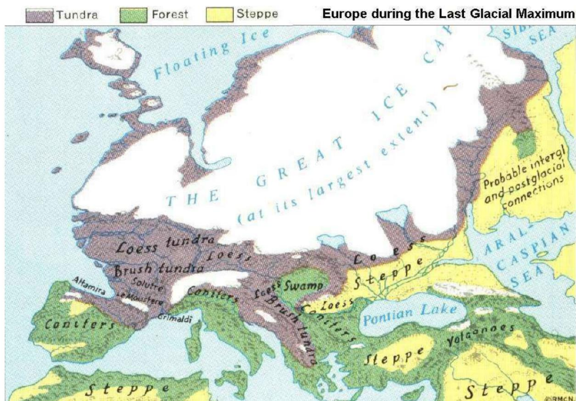
Figure 4. L'Europe lors du dernier maximum glaciaire, il y a environ 23 000 ans. Le niveau de la mer est plus bas d'environ -125 m, la végétation et l'habitat sont radicalement modifiés et l'extension de la calotte glaciaire est telle qu'elle recouvre la majeure partie de l'Europe continentale. Les mammouths de laine se trouvaient en Espagne et 80 % des terres arables ont été perdues par rapport à aujourd'hui.
